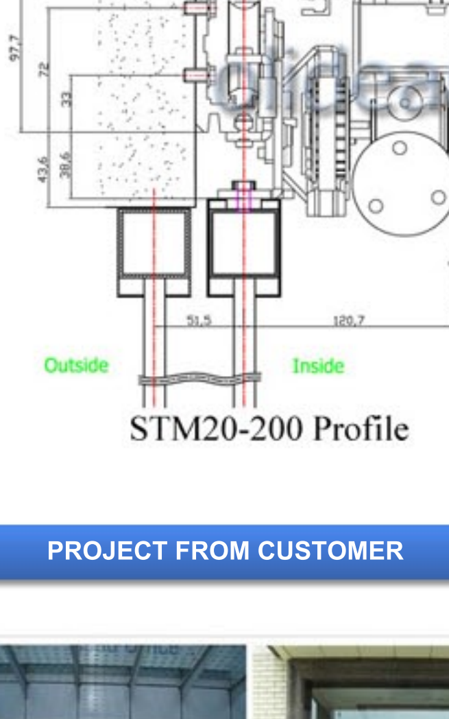
STM20-200 Profile
